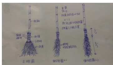
竹掃把的製作流程（手繪示意）
